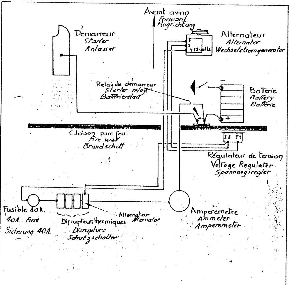
— Schéma de principe du circuit électrique —
